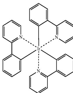
Ir(ppy) 3
