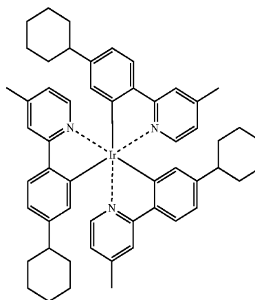
Ir(ppy) 3
