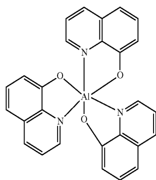
Alq 3
