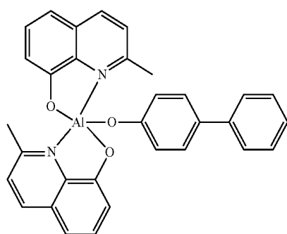
BAlq
