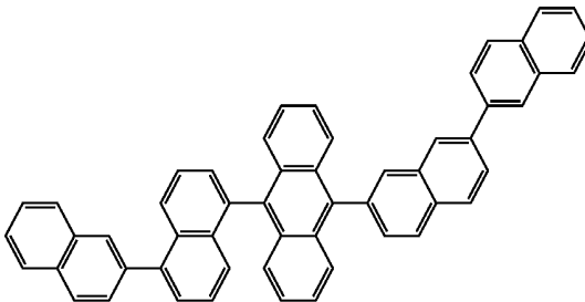
H17
