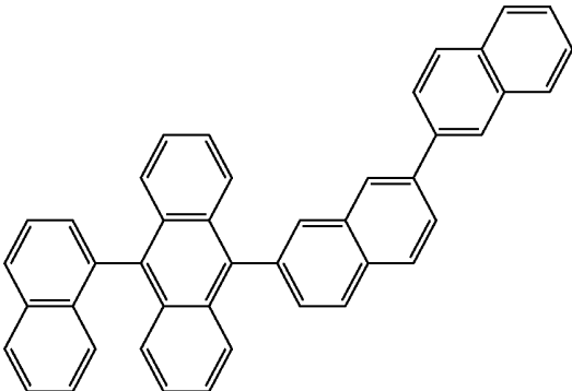
H18
